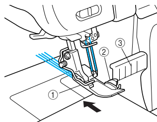
① Прижимная лапка ② Верхний нож ③ Шаблон припусков на швы
